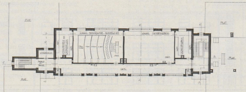
Tweede verdieping. Schaal 1 : 400.
