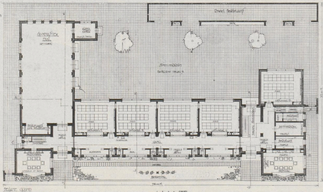
Begane grond. Schaal 1 : 400.
